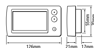
ST40 Dimensions
