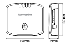
ST290 DPU Dimensions
