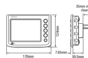
ST290 DPU Dimensions
