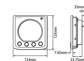
ST290 Keypad Dimensions
