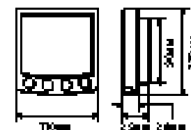
ST60 Plus Dimensions
